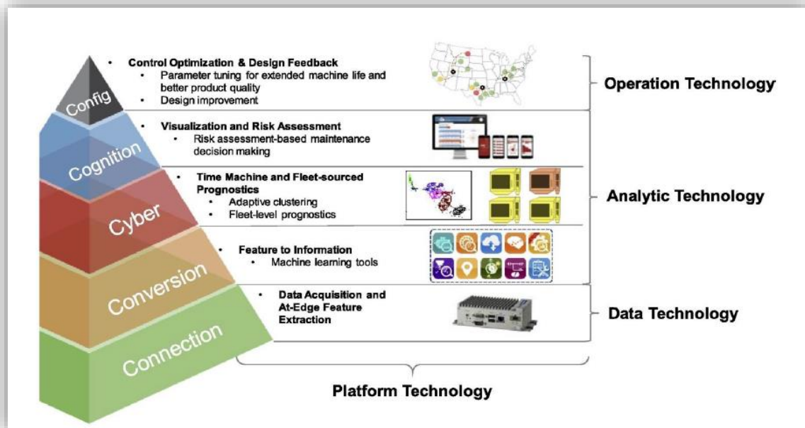
شكل رقم 01: تقنيات التمكين للذكاء الاصطناعي الصناعي
